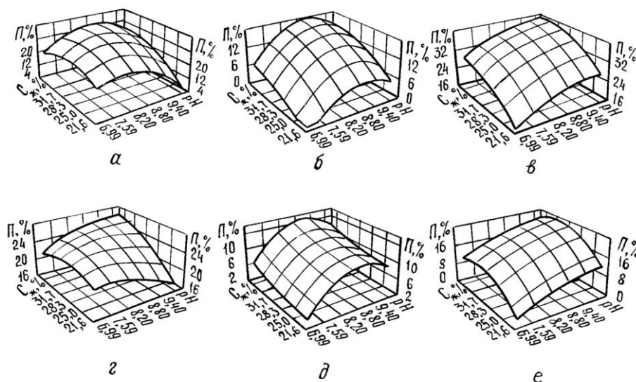
Рис. 4. Зависимость степени очистки P по ХПК ( a - в ) и БПК 5 ( d - e ) от условий получения образцов: a – ДМ, b – АИ, в – ГЛ
